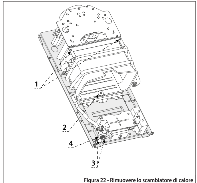
Figura 22 - Rimuovere lo scambiatore di calore
