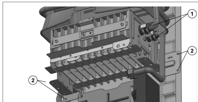
Figura 21 - Retire el quemador principal
