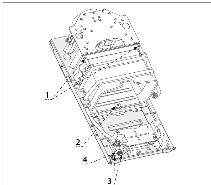
Figura 17 - Retirar el intercambiador de calor
