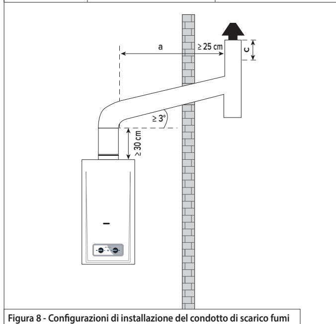
Figura 8 - Configurazioni di installazione del condotto di scarico fumi
