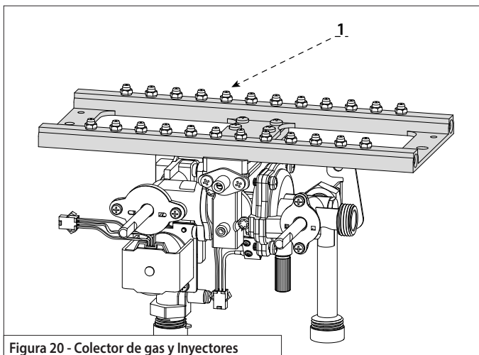
Figura 20 - Colector de gas y Inyectores
