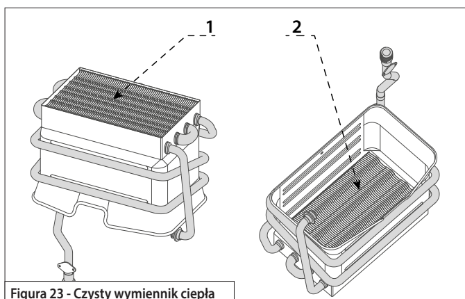
Figura 23 - Czysty wymiennik ciepła
