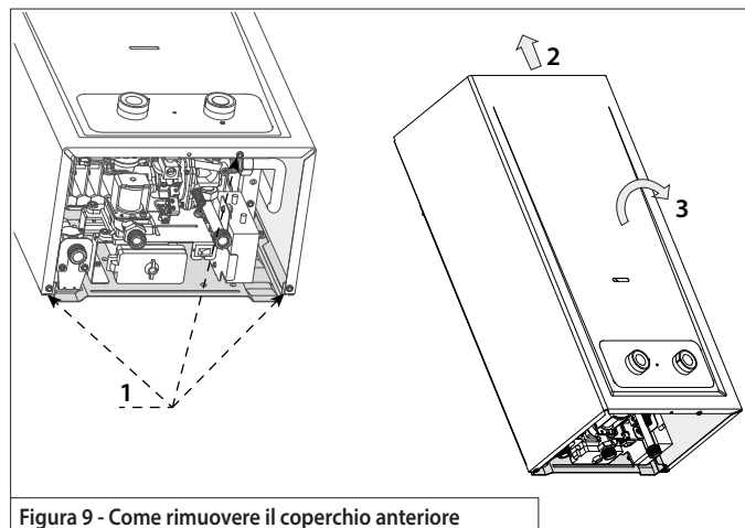
Figura 9 - Come rimuovere il coperchio anteriore
