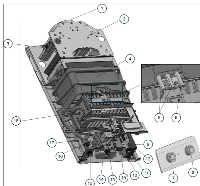
Figura 3 - Vista complessiva
