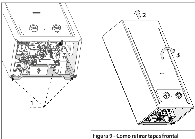
Figura 9 - Cómo retirar tapas frontal
