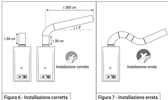
Figura 6 - Installazione corretta
