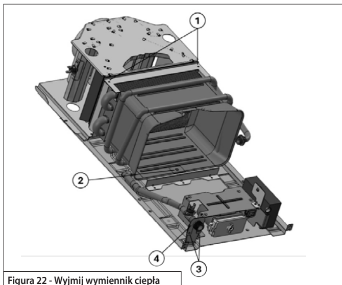
Figura 22 - Wyjmij wymiennik ciepła
