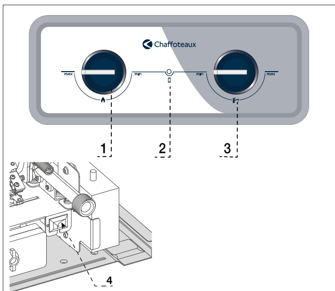
Figura 2 - Panel sterowania i przycisk włączania/wyłączania
