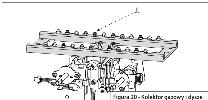
Figura 20 - Kolektor gazowy i dysze
