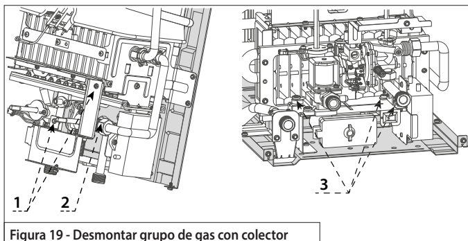
Figura 19 - Desmontar grupo de gas con colector
