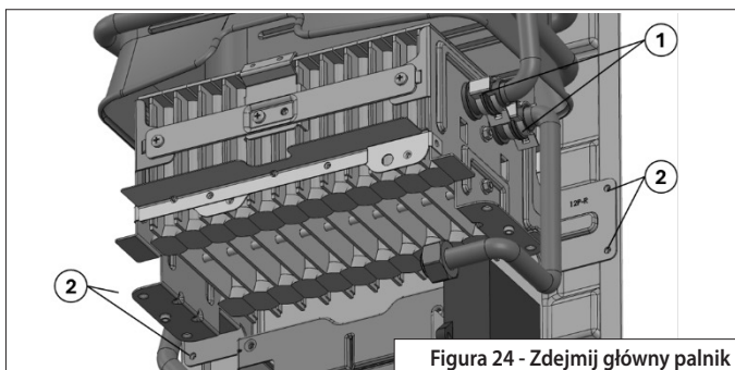
Figura 24 - Zdejmij główny palnik
