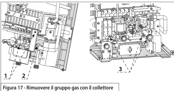
Figura 17 - Rimuovere il gruppo gas con il collettore
