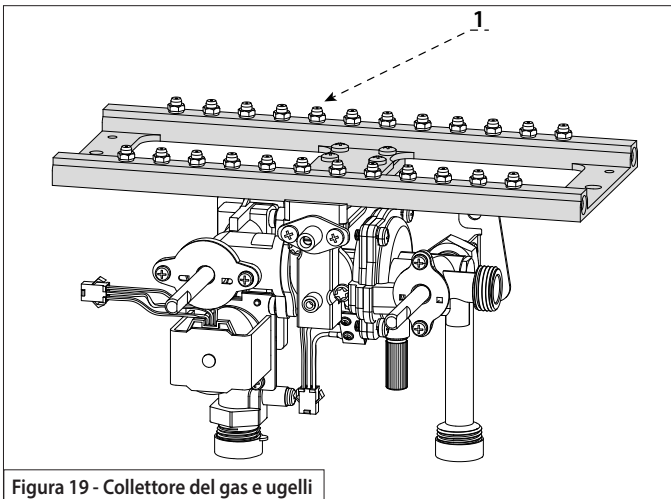
Figura 19 - Collettore del gas e ugelli
