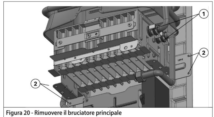
Figura 20 - Rimuovere il bruciatore principale
