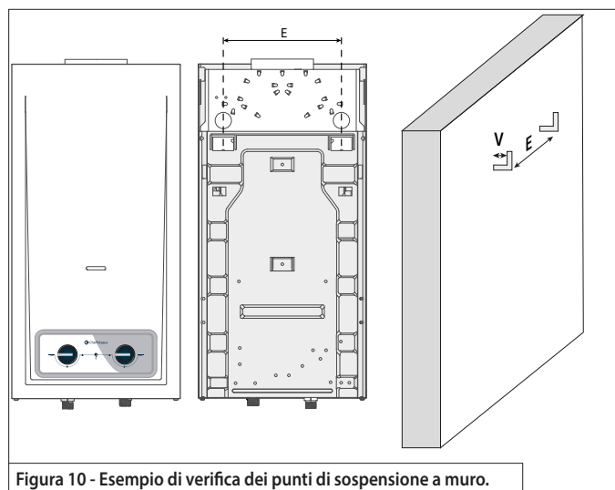
Figura 10 - Esempio di verifica dei punti di sospensione a muro.
