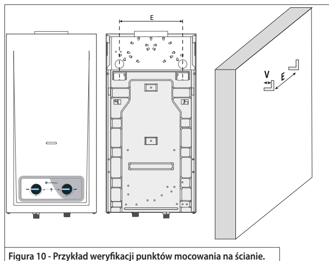
Figura 10 - Przykład weryfikacji punktów mocowania na ścianie.
